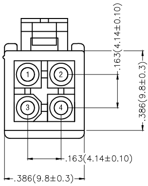
4 Circuits
