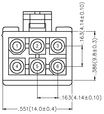
6 Circuits
